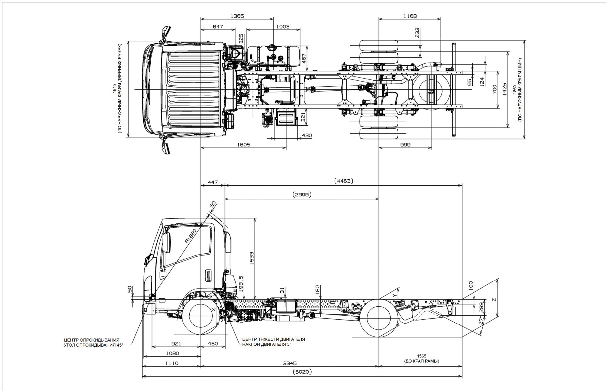
Рис. 9-1-3. Чертеж шасси с кабиной. NMR85L-НН5АУУ
